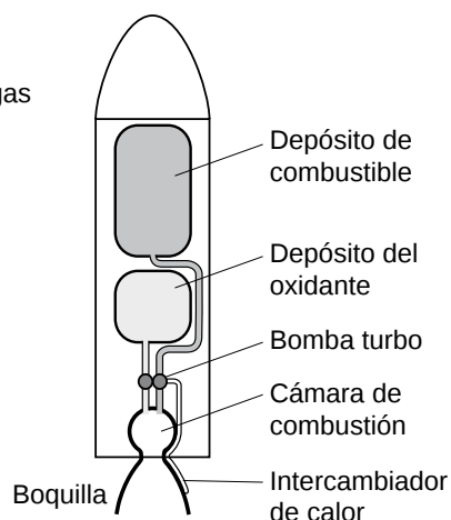
Cohete líquido (tipo bomba turbo)
