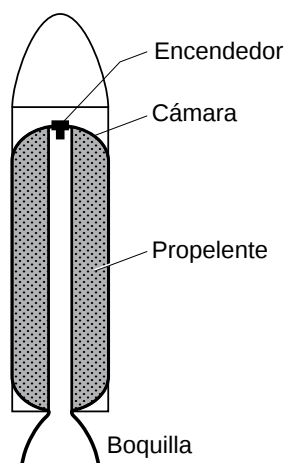
Cohete sólido
